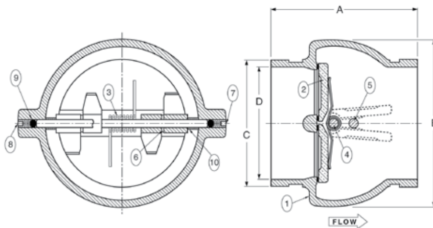
KG-900-W-LF Grooved
